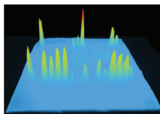
Výsledek při chlazení kamery na -25^{\circ}\text{C} 2-stupňový Peltier
